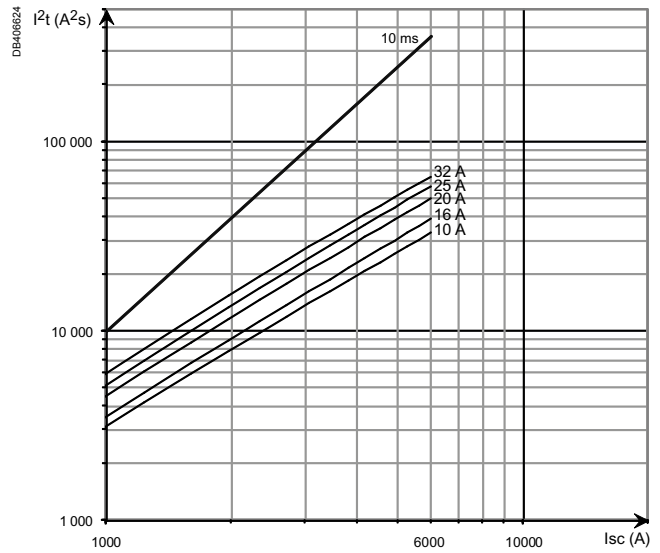
DCP N Vigi (4P - 400 V)
